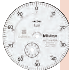
Graduación: 0.001mm Intervalo de medición: 1mm
