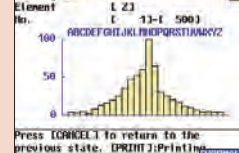
Resultado de la medición de perpendicularidad: Pantalla gráfica
