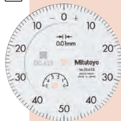
Graduación: 0.01mm Intervalo de medición: 5mm
