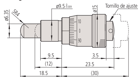
148-342 Peso: 29g
