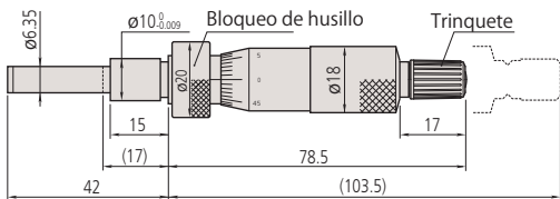
150-209
