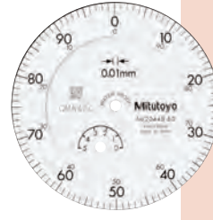
2044S-60 Tipo a prueba de agua
