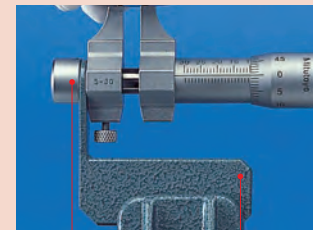
Tapa (No.300401) Sujetador (No.300400)
