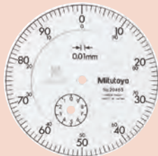
Carátula continua (Graduación bidireccional)
