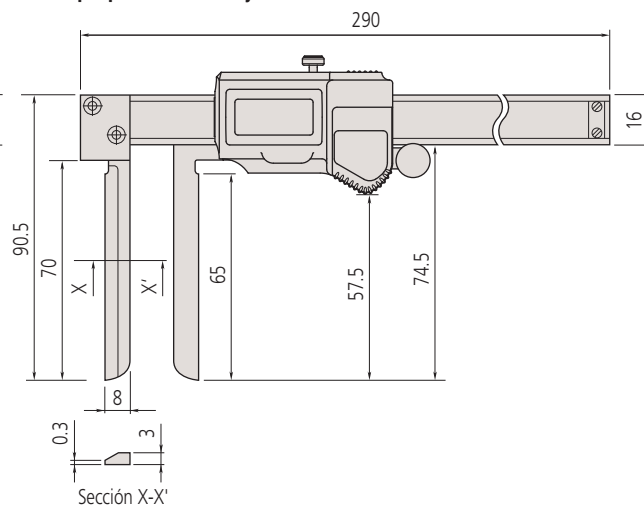
Tipo punta de navaja: 573-642, 643, 742
