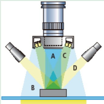
A: Iluminación vertical de superficie (Halógena)
