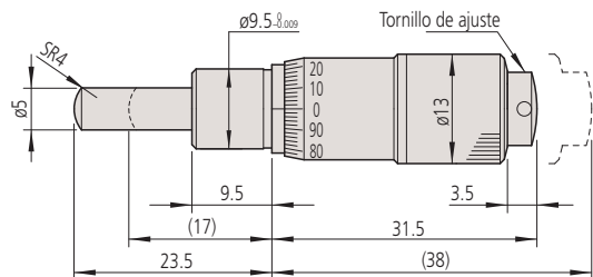
148-142 Peso: 31g
