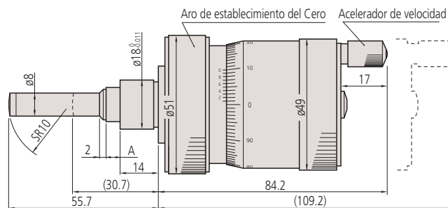
152-402
