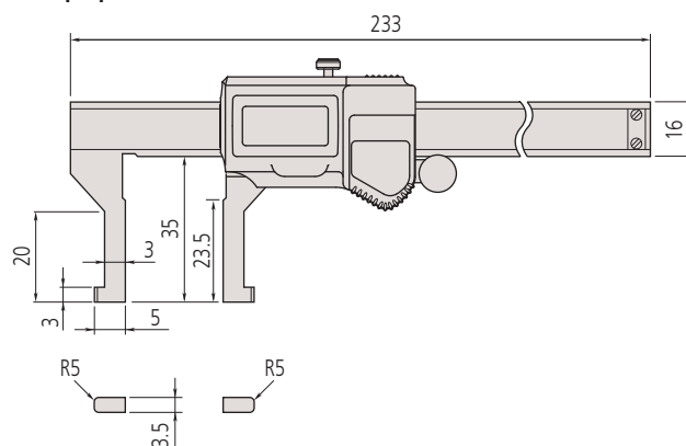
Tipo para ranura interior: 573-645, 647, 745
