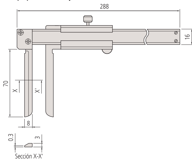
Tipo punta de navaja: 536-142
