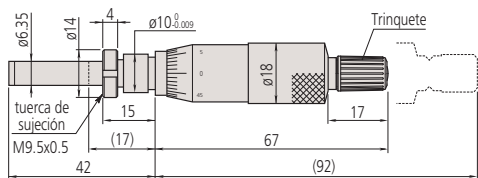
Esesor accesorio: 11.5mm 150-191
