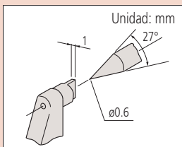
142-402, 142-403
