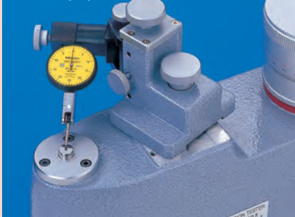
Calibrando un indicador de caratula tipo palanca
