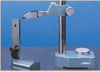
Fijando un indicador de carátula tipo palanca a un apilamiento de bloques patrón sujetados a la base con un conector tipo D
