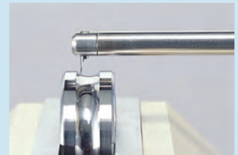
Contorno interior y exterior de un cojinete
