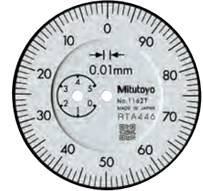
Graduación: 0.01mm Intervalo de medición: 5mm
