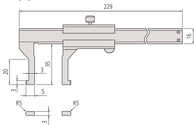
Tipo para ranura interior: 536-145
