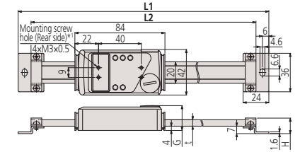
SDV-E (450 hasta 1000mm) / SDV-F (450 hasta 1000mm)
