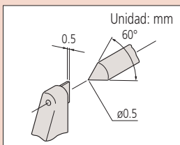
342-271, 342-371, 112-401
