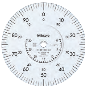
Graduación: 0.01mm Intervalo de medición: 30mm 3052S-19
