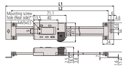
SDV-E (hasta 300mm) / SDV-F (hasta 300mm)
