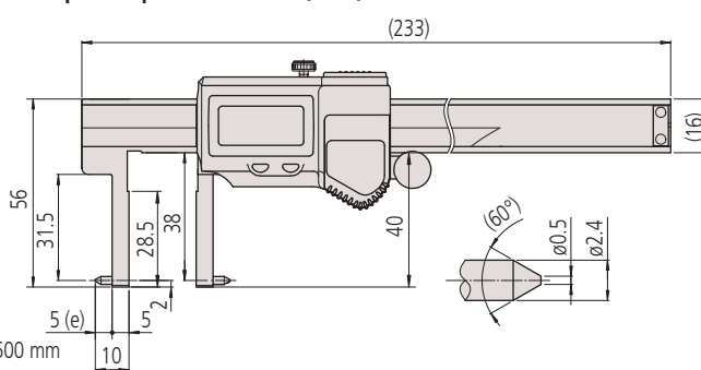
Tipo con puntas: 573-646, 648, 746
