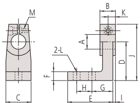
(Unidad: mm)
