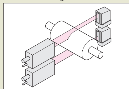
Sistema dual para medición de un diámetro exterior grande
