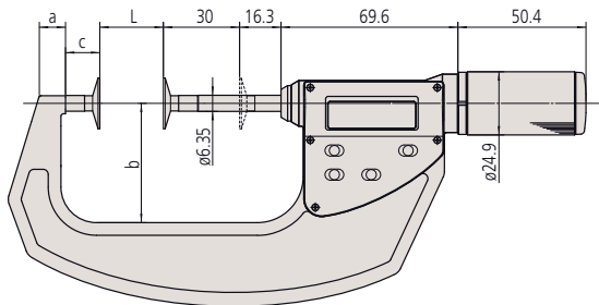
Tipo Quickmike
