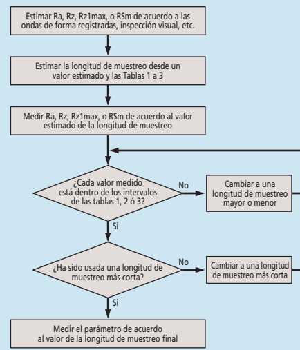
Fig.1 Procedimiento para determinar la longitud de muestreo de un perfil no periódico si no se especifica
