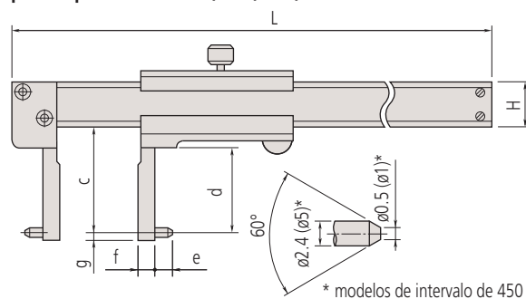
Tipo con puntas: 536-146, 147, 148, 149
