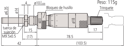
Esesor accesorio: 11.5mm 150-210
