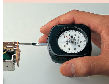
Medición de la fuerza de contacto en un relé
